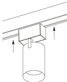
Рис. 2. Установка светильника
