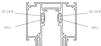
Рис. 4. Расположение контактов на шинопровode
