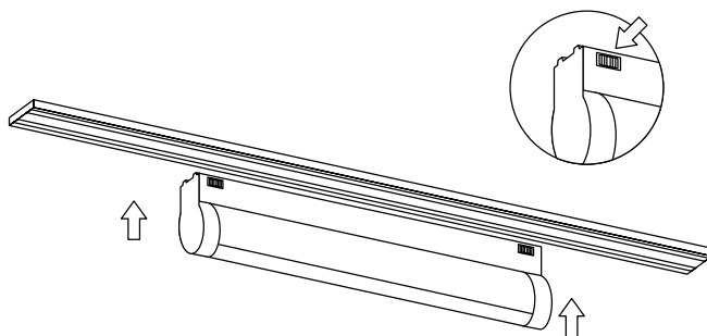
Рис. 2. Установка светильника
