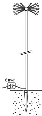
Рис. 2. Установка светильника в грунт
