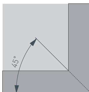
Рис. 1. Распил профиля ①. Вид сверху
