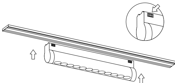
Рис. 2. Установка светильника
