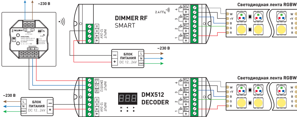
Рис. 1. Схема подключения панели управления
